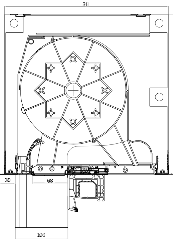
SKB Styroterm 300 ispezione esterna
