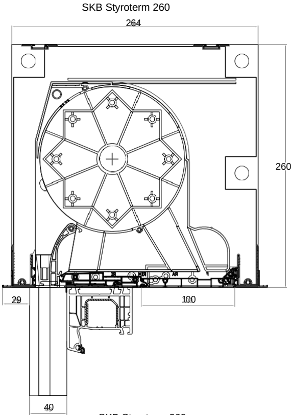
SKB Styroterm 260 ispezione esterna
