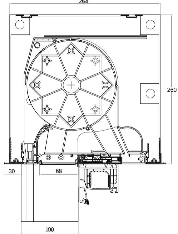
SKB Styroterm 260 ispezione esterna
