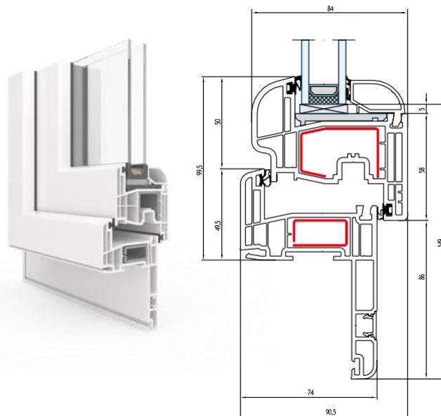
RISTRUTTURAZIONE 64,5 MM
