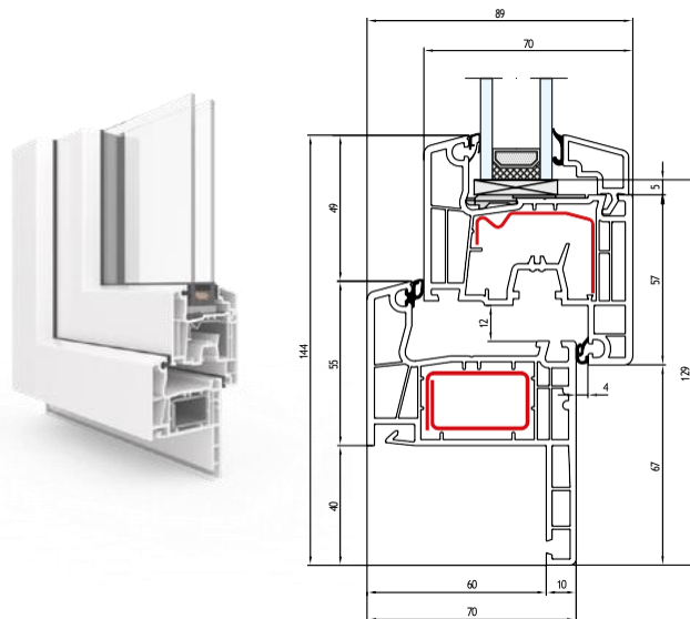
RISTRUTTURAZIONE 40 MM
