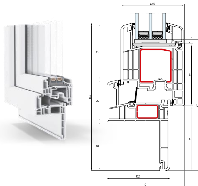
RISTRUTTURAZIONE 60 MM
