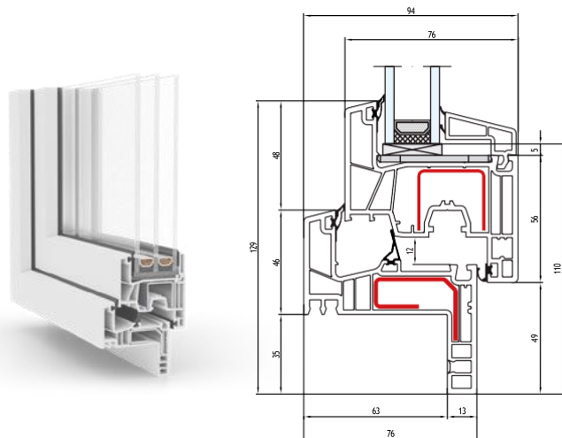
RISTRUTTURAZIONE 35 MM
