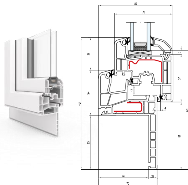
RISTRUTTURAZIONE 65 MM
