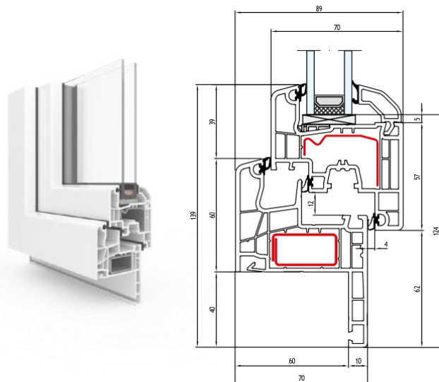
RISTRUTTURAZIONE 40 MM
