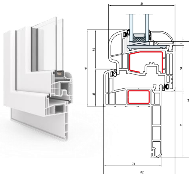
RISTRUTTURAZIONE 65 MM
