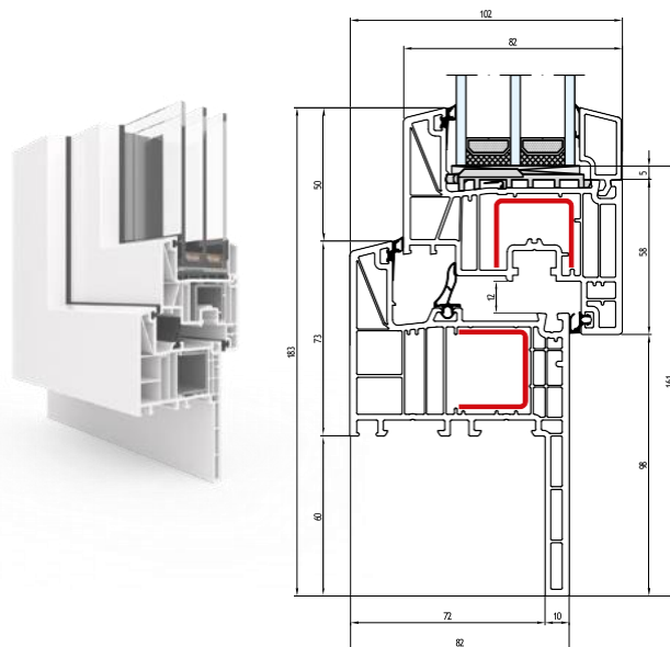
RISTRUTTURAZIONE 60 MM
