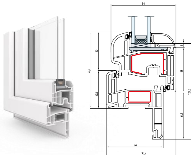
RISTRUTTURAZIONE 40 MM
