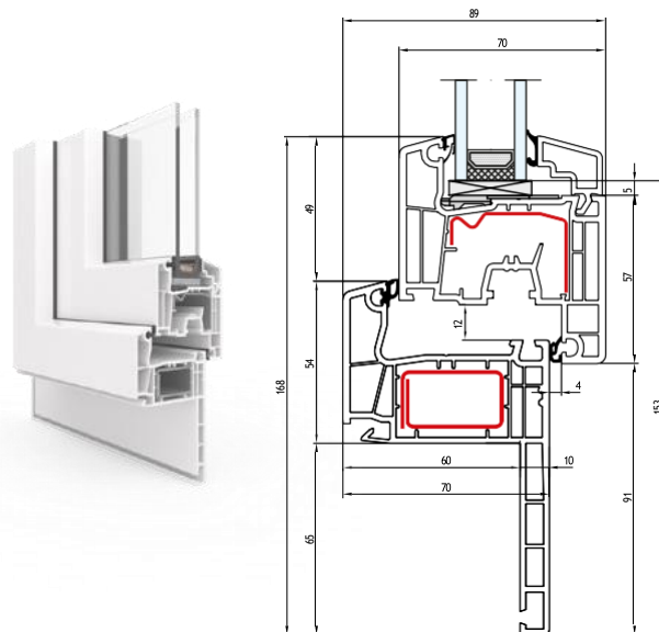
RISTRUTTURAZIONE 65 MM
