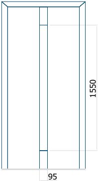
Disegno tecnico
